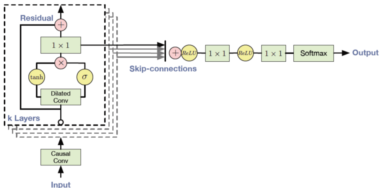
Рис. 5: Архитектура WaveNet
