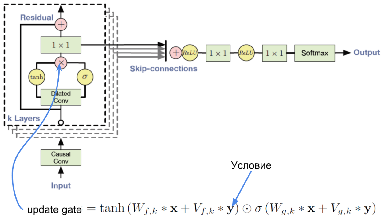
Рис. 7: Gate, отвечающий за условия
