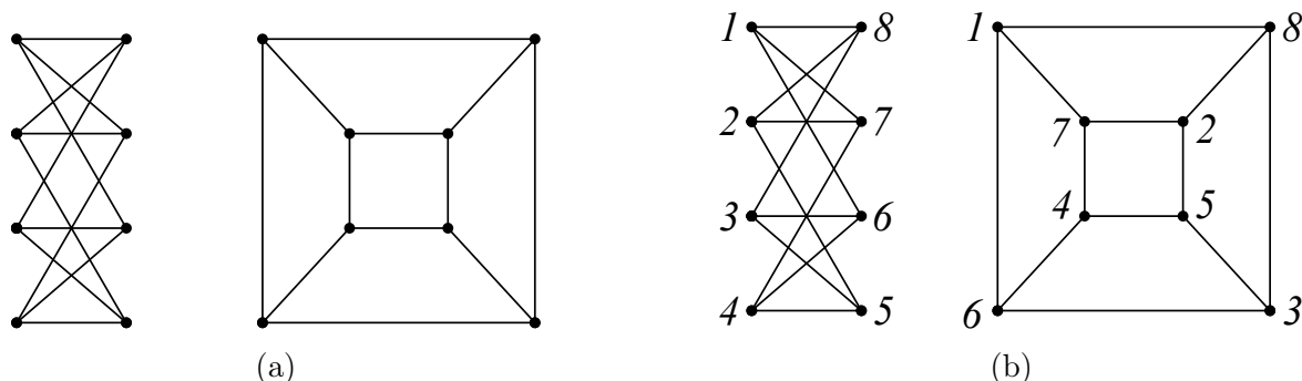
Рис. 25: Установление изоморфизма между графами
