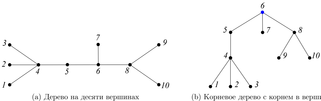
Рис. 30: Дерево и корневое дерево
