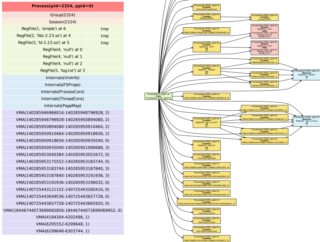
Рис. 2.3: Дерево из одного процесса и граф действий восстановления для него
